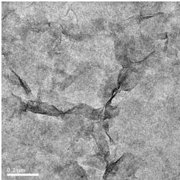
MoS 2 Nanosheet
