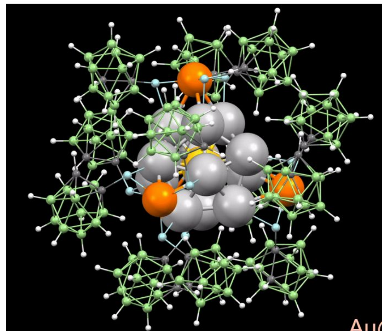
Au@Ag 16
